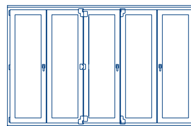
Esquema 532
