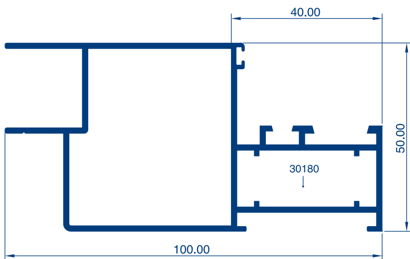
Ref. 2056 Espesor 1.5
