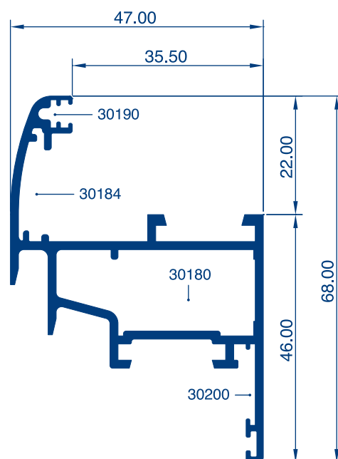
Ref. 2042 Espesor 1.5
