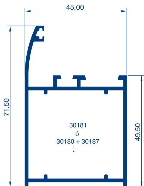
Ref. 2066 Espesor 1.5
