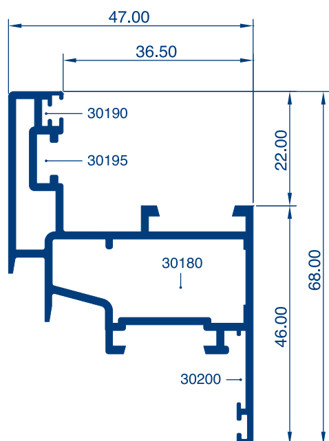
Ref. 2010 Espesor 1.4
