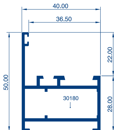
Ref. 2041 Espesor 1.5
