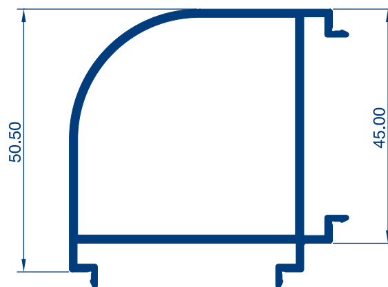
Ref. 2131 Espesor 1.5
