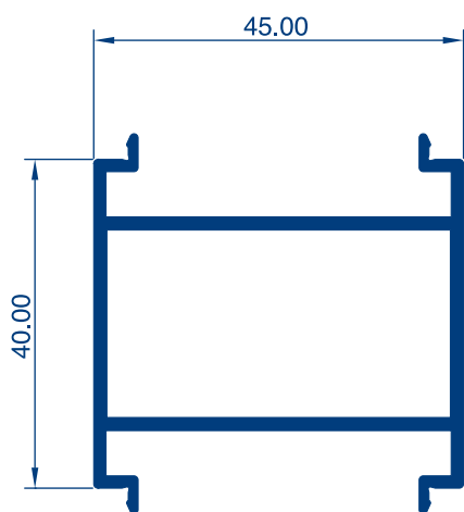
Ref. 2130 Espesor 1.5
