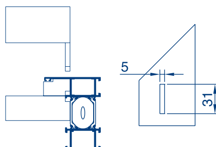
7.- MECANIZADO DESAGÜE DE MARCO.
